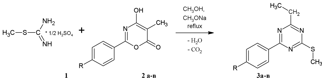
Рисунок. Синтез новых производных 1,3,5-триазины где: R = NO 2 , (а) H, (б) CH 3 (в)
