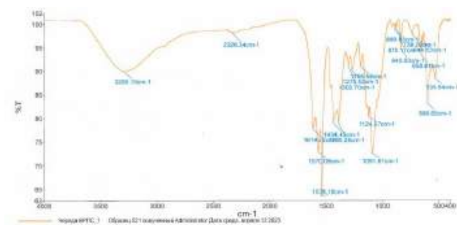
Рис. 2. ИК-спектр водорастворимых полисахаридов Bidens frondosa L.
