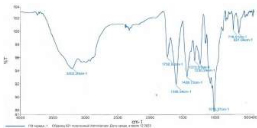
Рис. 3. ИК-спектр пектиновых веществ Bidens frondosa L.
