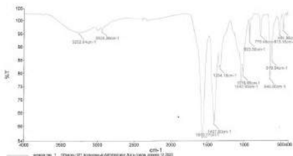
Рис. 4. ИК-спектр гемицеллюлоз Bidens frondosa L.
