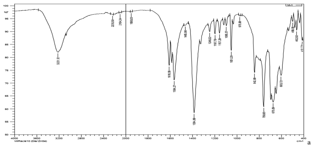
Рисунок 2. ИК спектры ГЛК (а), 3-ПМК(б), Na(3-ПМК-Н) (в)
