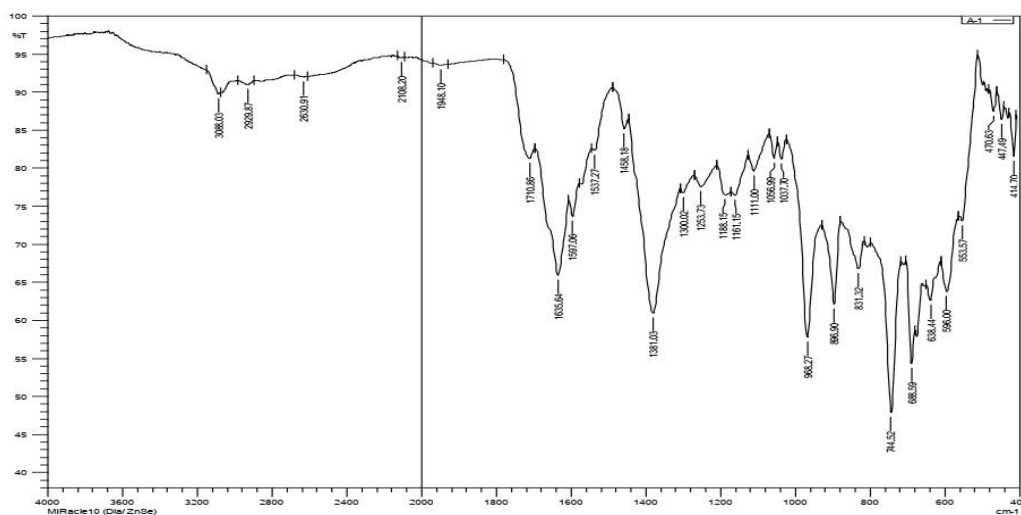
Рисунок 3. ИК спектры \text{Co}(\text{ГЛК-2H})(3\text{-ПМК})\cdot 2\text{H}_2\text{O} (а), \text{Ni}(\text{ГЛК-2H})(3\text{-ПМК})\cdot 3,5\text{H}_2\text{O} (б), \text{VO}(\text{ГЛК-2H})(3\text{-ПМК})\cdot \text{H}_2\text{O} (в)
