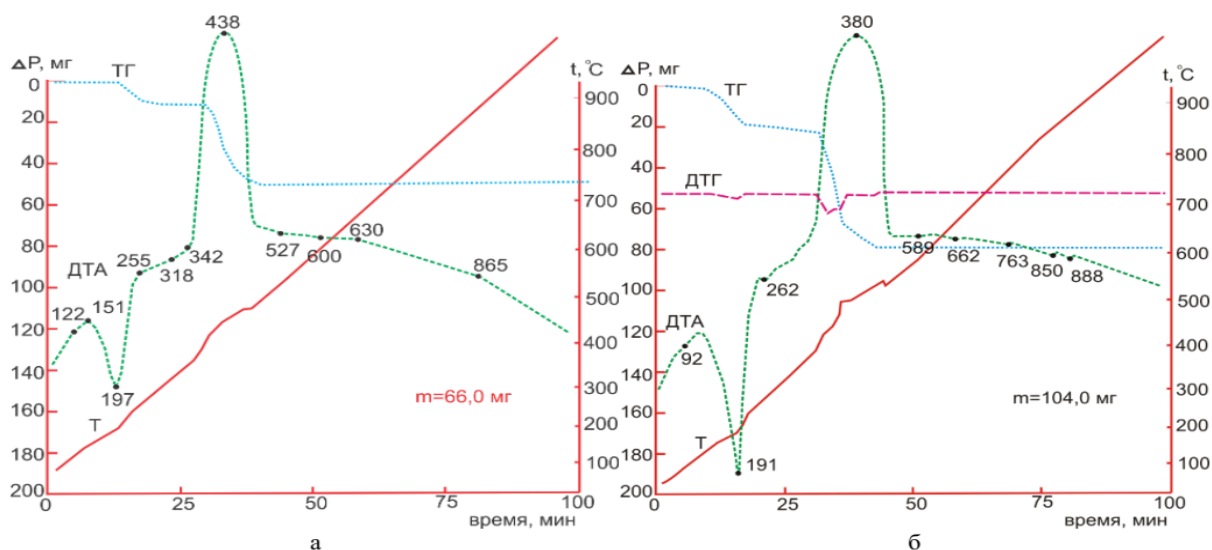
Рисунок 4. Дериватограммы Ni(ГЛК-2H)(3-ПМК)·3,5H 2 O (а), Co(ГЛК-2H)(3-ПМК)·2H 2 O (б)
